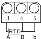
●K、J、E、R、S、B、T配線圖
